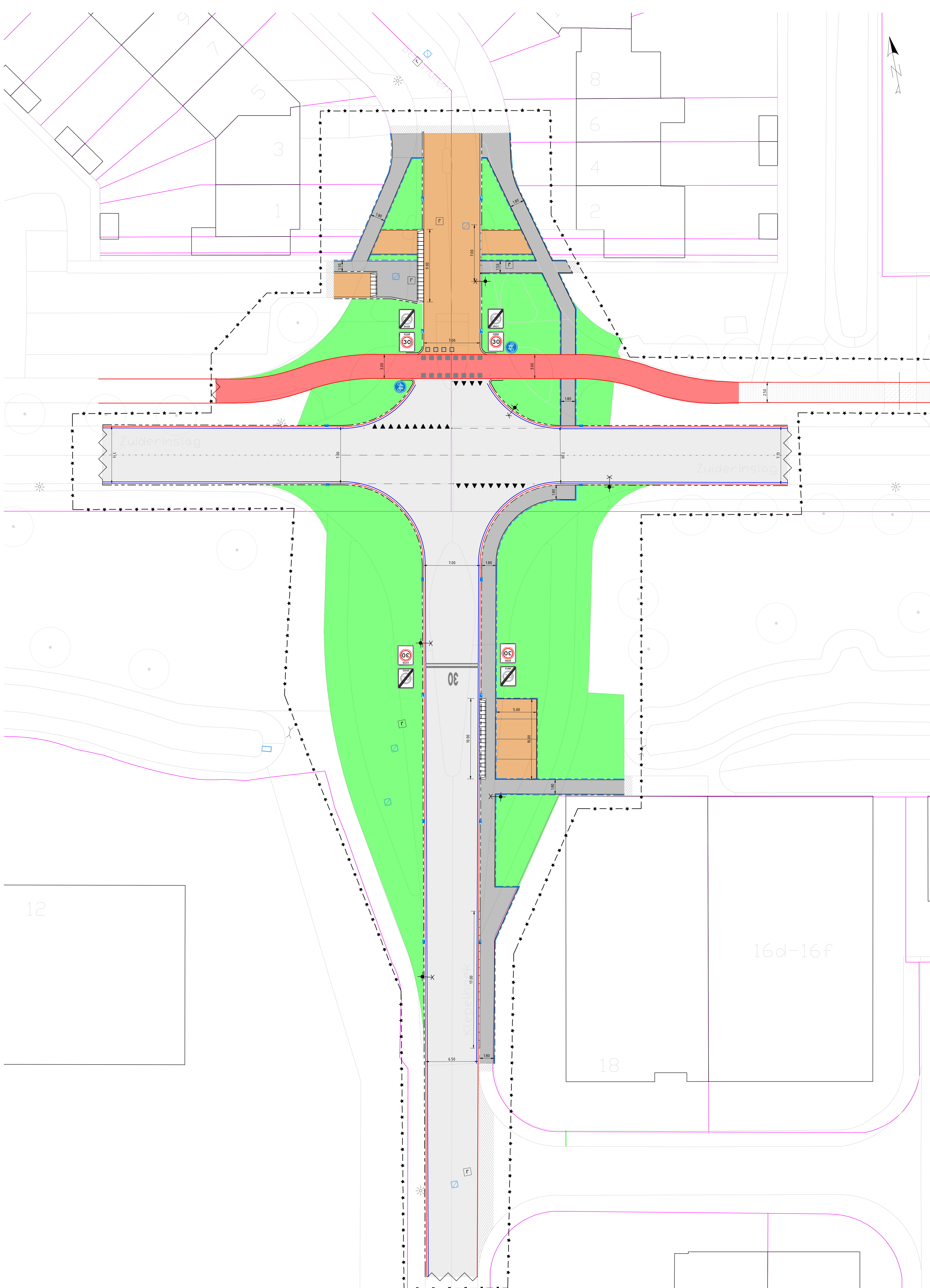
Nieuwe situatie Schaal 1:200
