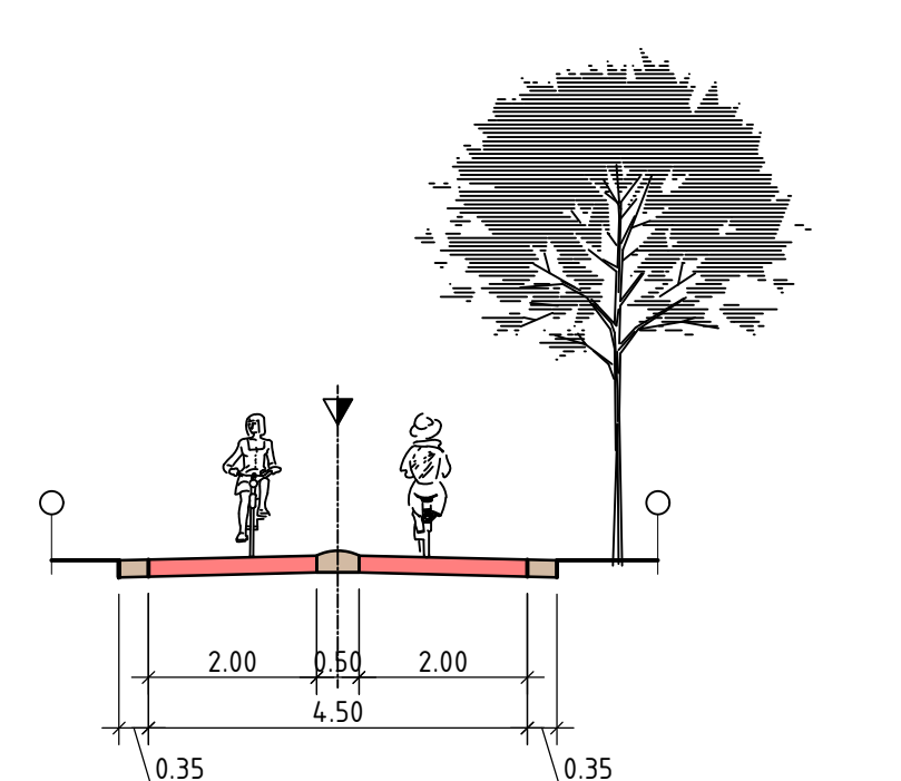
DOORSNEDE 3 SCHAAL 1:100
