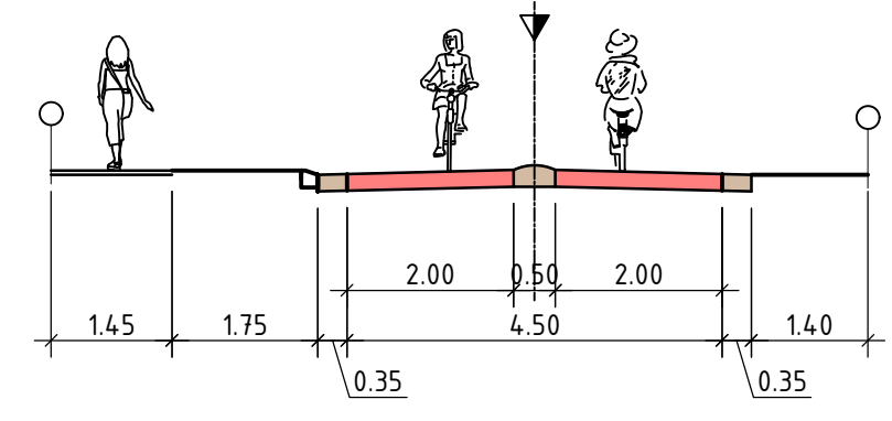
DOORSNEDE 1 SCHAAL 1:100
