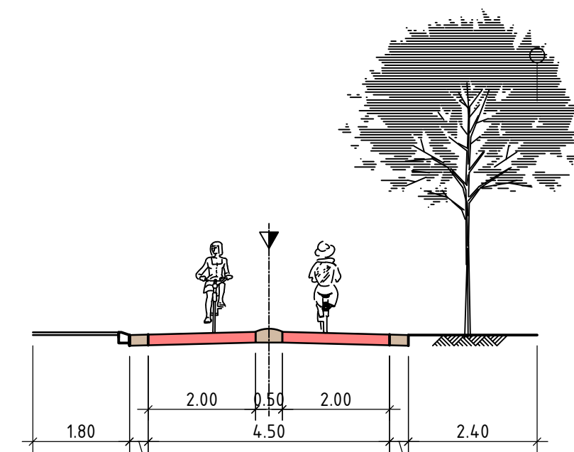
DOORSNEDE 2 SCHAAL 1:100
