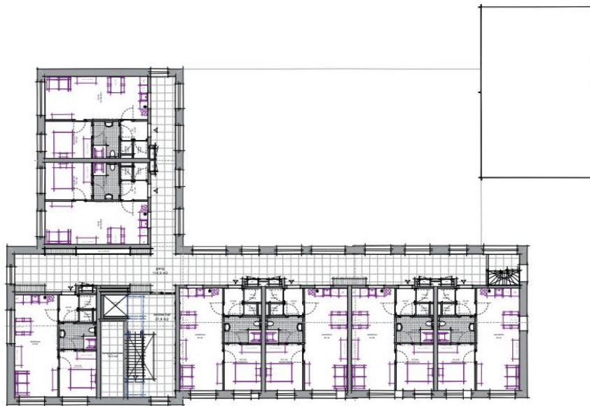
1e verdieping
