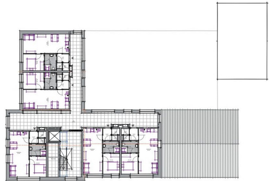
2e verdieping
